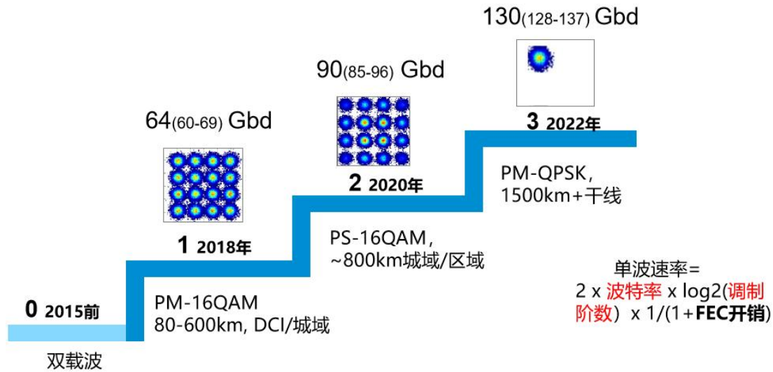
图 1.4. 单波 400G 系统主要特征及传输能力
