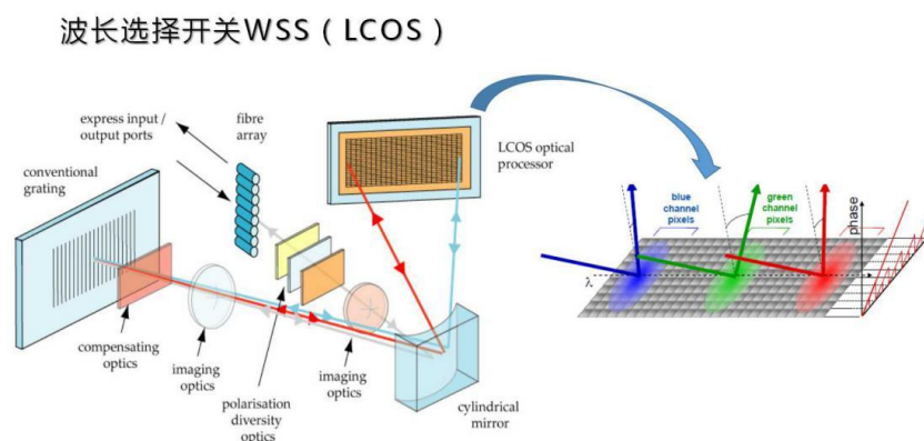
图 2.5 波长选择开关 WSS (LCOS) 结构原理
